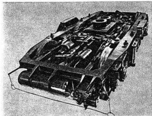
Eines der neuen dreiaxigen Mitteldrehgestelle für die Doppelstockgliederzüge.
