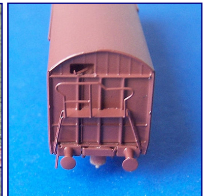
Der gedeckte Wagen Gbs 150 skandinavischer Staatsbahnen (Bild links) erscheint ebenfalls 2012 bei FR. Eine Besonderheit seines Vorbilds ist die Bremserbühne mit der in die Stirnwand ragenden Handbremskurbel. Beide Fotos: FR Freudenreich Feinwerktechnik
