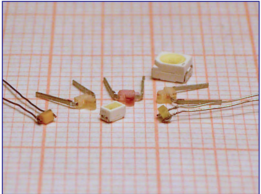
Bei SMD-Leuchtdioden (im Bild insgesamt vier Exemplare mit und ohne angelötete Drähte) ist es häufig sehr schwierig, Markierungen zur korrekten Polung zu erkennen.
