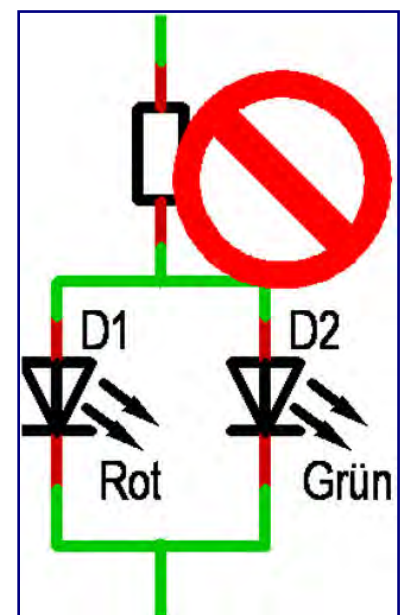
Abbildung 4 (rechts): Das geht nicht! Die rote Leuchtdiode hat eine geringere Flussspannung als die grüne, die dann gar nicht leuchtet.
