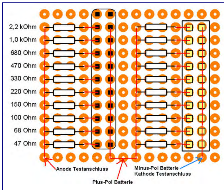
Abbildung 9: So können die wenigen Bauelemente verdrahtet werden. Die roten Striche sollen Verbindungen auf der Lötseite darstellen. Die elfte, offene Position des Jumpers ist die Aus-Stellung, damit er nicht verloren geht.
