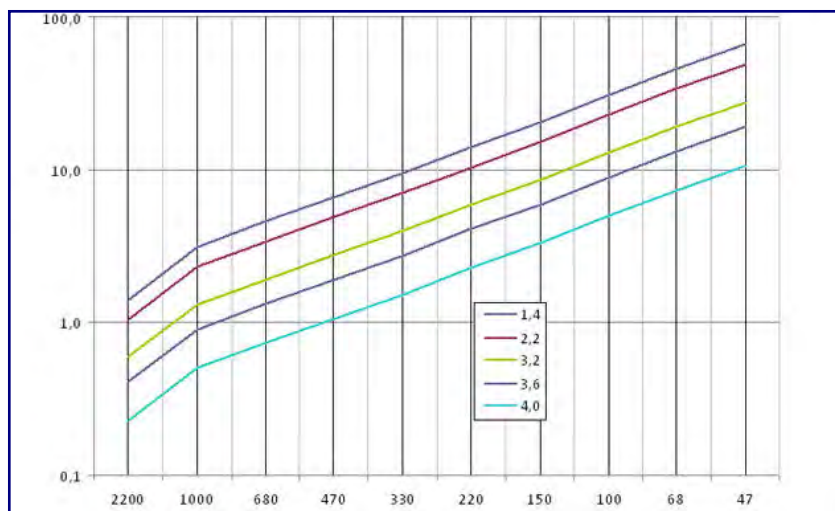
Abbildung 3: Je nach Typ bzw. Flussspannung einer LED und der Versorgungsspannung (Y-Achse, Maßeinheit V) sind unterschiedliche Widerstände zu wählen (X-Achse, Maßeinheit Ohm), um einen gewünschten Strom einzustellen (farbige Kennzeichnung der Betriebsspannung in V).
