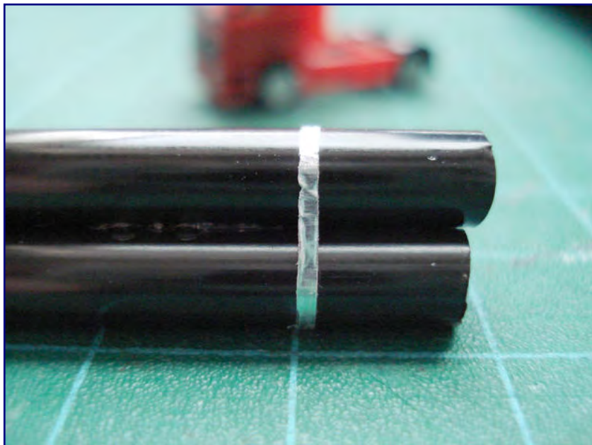
In der Makroaufnahme zeigt sich die gute Wirkung des Aluminium-Klebebands. Soweit möglich, sollten im Modell immer die Originalwerkstoffe oder zumindest sehr ähnliche zum Einsatz kommen, wie diese Aufnahme lehrt.
