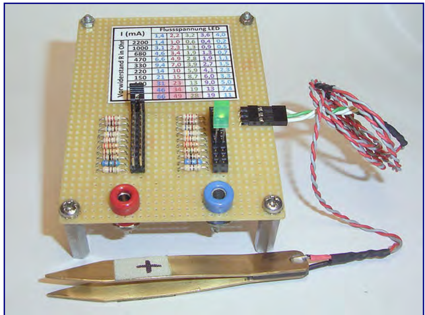
Schon wenige Bauteile können ein praktisches Testgerät für Experimente mit Leuchtdioden ergeben.
