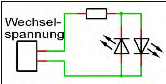
Abbildung 5 (oben): Eine Diode hält die negative Spannung von einer LED fern. So ist auch der Betrieb an einer Wechselspannung möglich.
