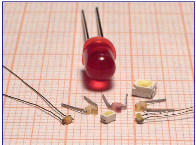
Ein Klassiker in Form einer roten 5-mm-LED neben verschiedenen SMD-Ausführungen und Miniaturleuchtdioden konventioneller Bauform. Dem Größenvergleich dient das Millimeterpapier als Unterlage.
