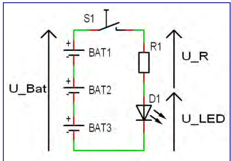
Abbildung 1: Prinzip-Schaltung zum Betrieb einer LED
